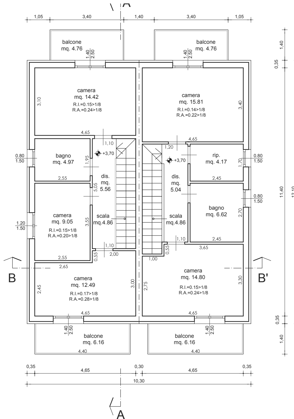
PIANO PRIMO
